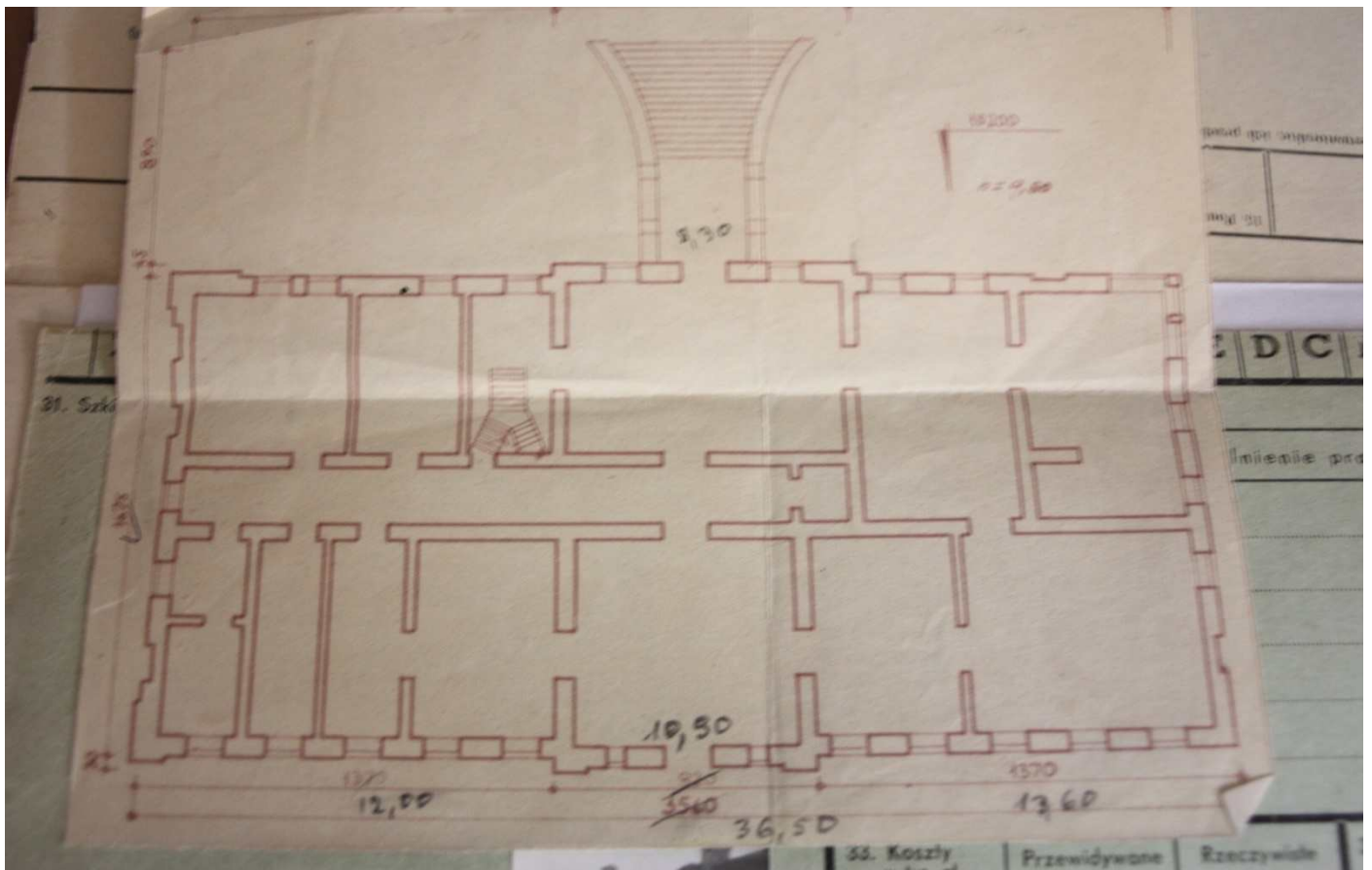
Plan ogólny pomieszczeń wraz z głównymi wymiarami budynku
